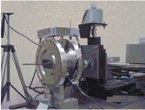
इण्डस-2 में इलेक्ट्रॉन किरण दिशा निर्धारक यंत्र
